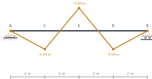
각 구간에서 직선적으로 변하는 휨모멘트도
