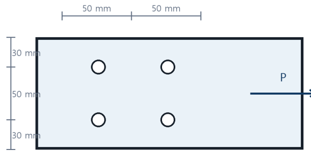
F10T-M20 표준구멍 · 판 두께 6 mm
