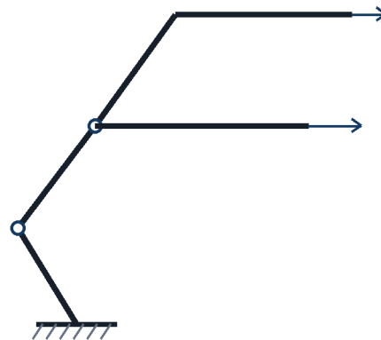
고정단과 두 내부힌지를 가진 골조
