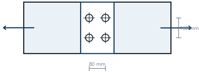
4-M22(F10T), PL-16 단순 인장접합
